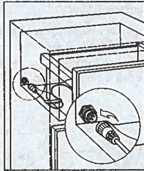
Cable de control (modelos de cajón)
